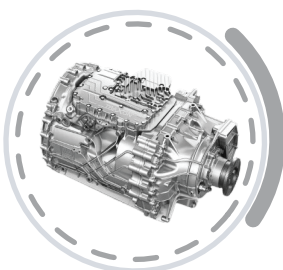
Transmisión Automatizada de 12 velocidades para trabajo pesado. ZF TRAXON AMT
